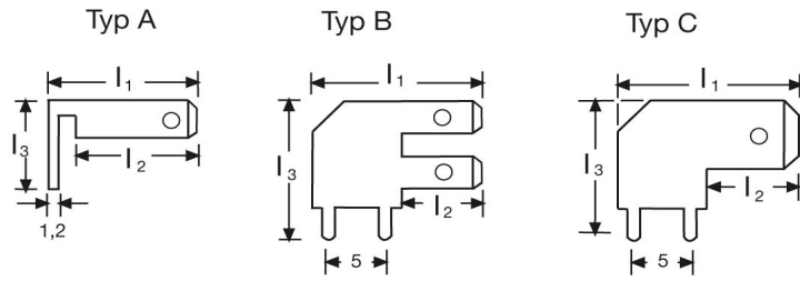
Flachstecker A,B,C abgewinkelt
